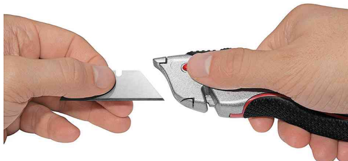
Safety-Cutter Profi Plus, Entriegelungsknopf zum Klingentausch
