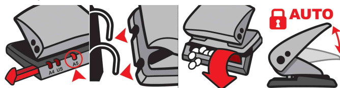
Réglette - système de centrage - réservoir à confettis à charnière - verrouillage du levier
