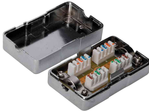
Verbindungsmodul Kat. 6 für Twisted Pair Kabel
