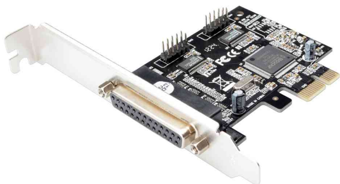
MCS9901 SPP/EPP/ECP PCI-Express série / parallèle, 2 ports séries / 1 port parallèle
