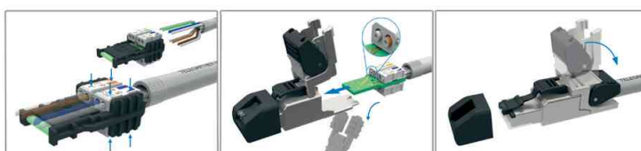
Connecteur Rj45 MFP8
