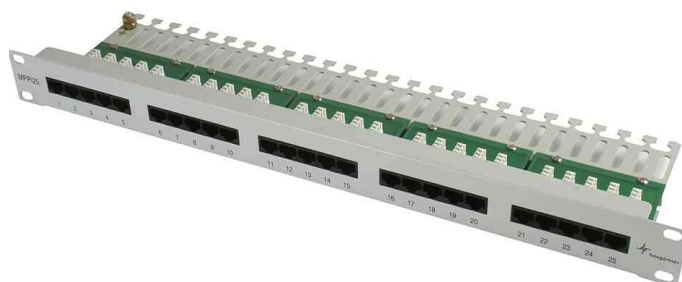
Panneau de brassage 19" RNIS sans gestion de brins
